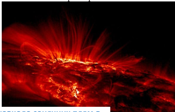
Рис. 3. Петлі навколо сонячних плям в ультрафіолеті, що демонструють потужні конвективні рухи в атмосфері Сонця. Спалахи зір типу UV Kuma мають так ж природу.
