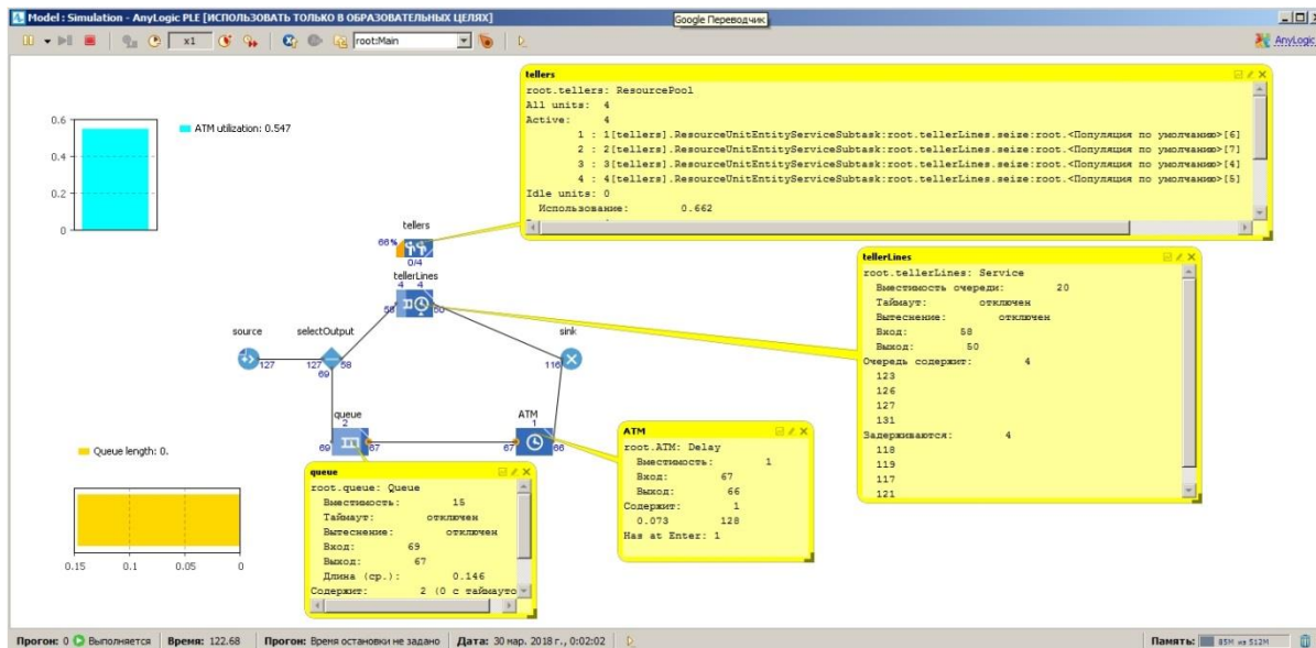
Рис.1. Імітаційна модель банку
