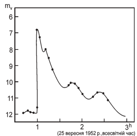
Рис. 2. Крива зміни блиску у спалаху зорі UV Кита
