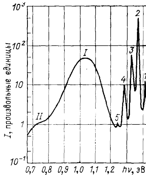
Рис.3. Спектр фотолюмінесценції InP при 6 К
