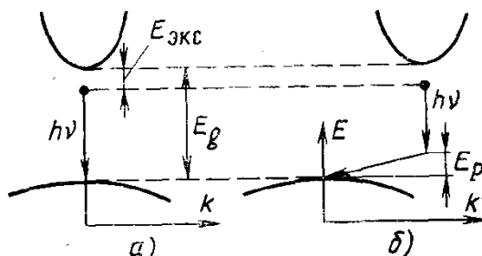
Рис.1. Екситонна рекомбінація: а – пряма; б – непряма
