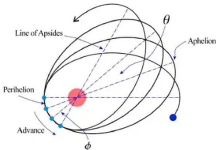
Рис.1 Прецесія перигелію
