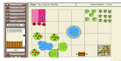
Рис. 5. Вікно програми
