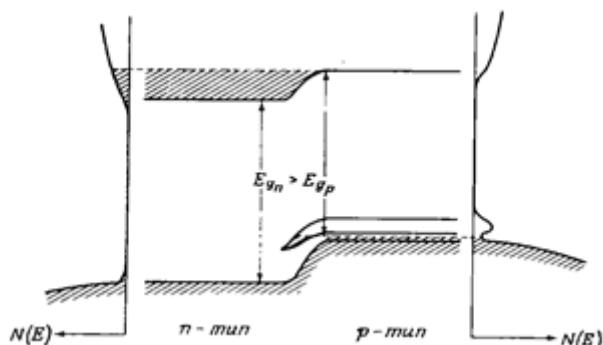
Рис. 2. Зміщений у прямому напрямку р - n – перехід, в якому викликане легуванням ефективне звуження ширини забороненої зони у р – області більше, ніж в n – області
