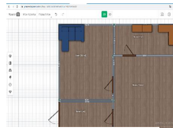
Рис. 3. Вікно програми
