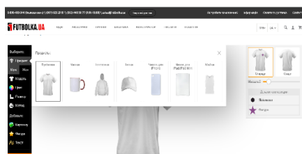
Рис. 4. Вікно програми
