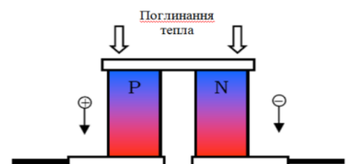
Рис. 5. Схема поглинання і випромінювання енергії на контактах двох напівпровідників
