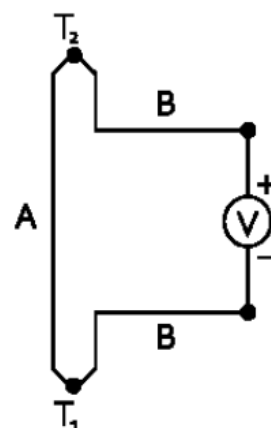
Рис. 1. Принципова схема ефекту Зеєбека
