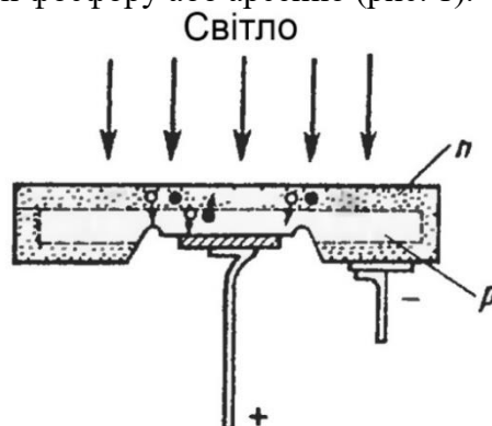
Рис. 1. Структура кремнієвого елемента
