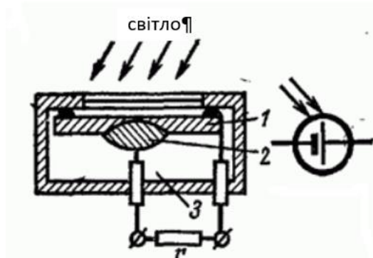
Рис. 1. Германієвий фотоелемент
