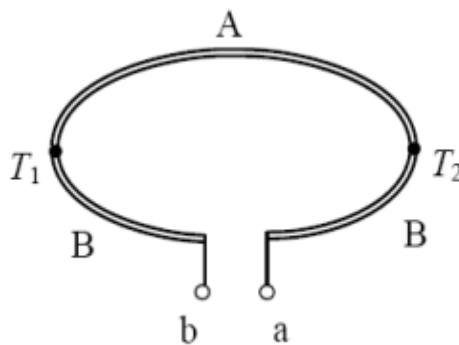
Рис. 3. Ефект Зеєбека у розімкнутому колі. a і b – два розімкнуті кінці кола
