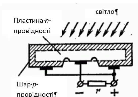
Рис. 2. Кремнієвий фотоелемент
