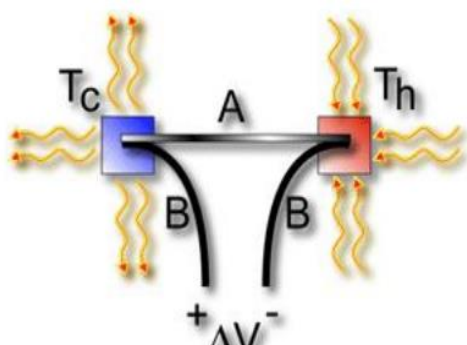
Рис. 2. Різниця потенціалів, V , яка виникає на розімкнутому кінці кола, що складається із двох різнорідних металів A і B , місця контакту яких знаходяться при різних температурах, прямо пропорційна різниці між гарячою та холодною температурами переходу T_h - T_c
