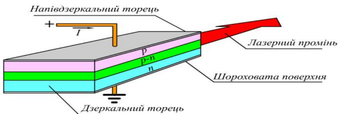
Рис.1 Будова напівпровідникового лазера [2]
