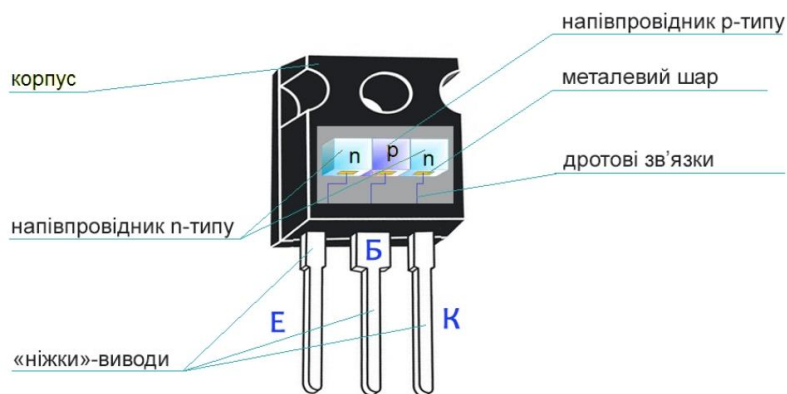
Рис. 2. Будова біполярного транзистора типу n-p-n
